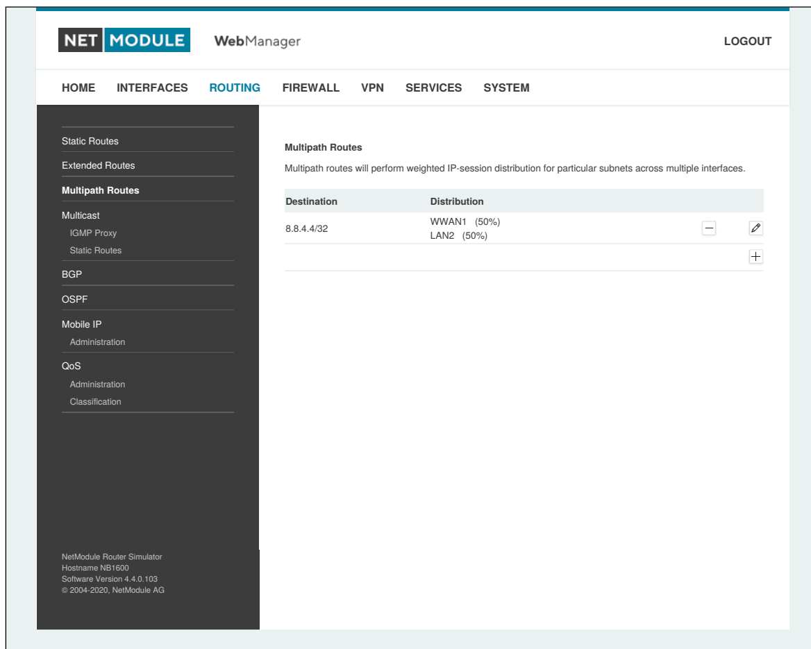
Abbildung 5.26.: Multipath-Routing
