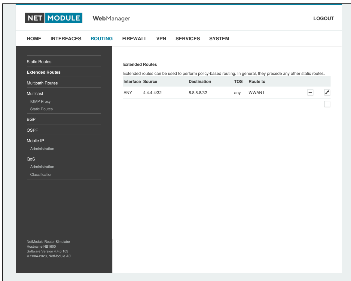
Abbildung 5.25.: Erweitertes Routing
