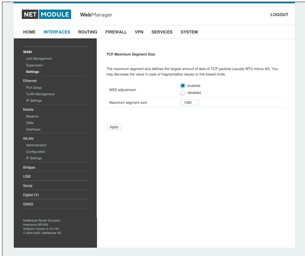
Abbildung 5.5.: WAN-Einstellungen
