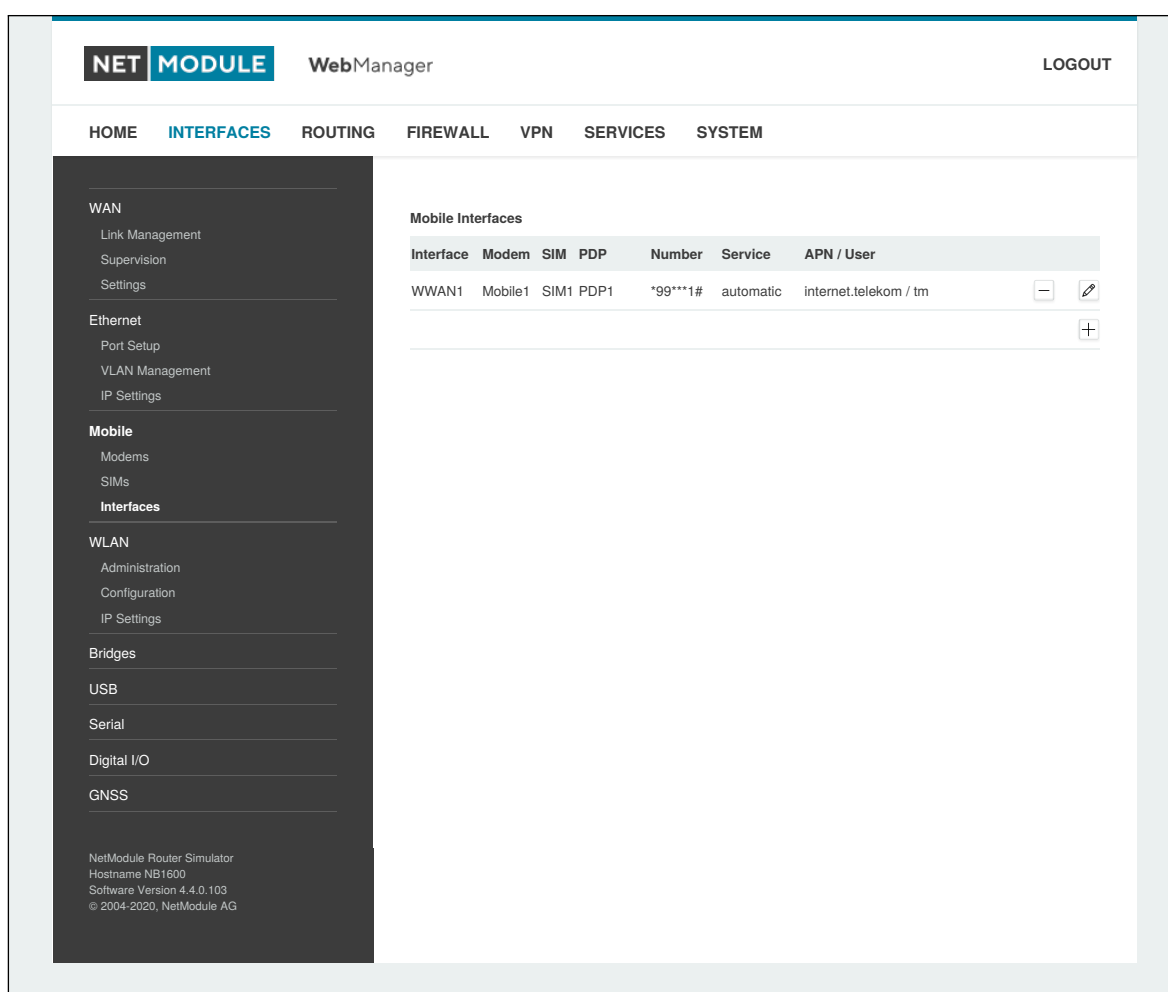
Abbildung 5.15.: WWAN-Schnittstellen
