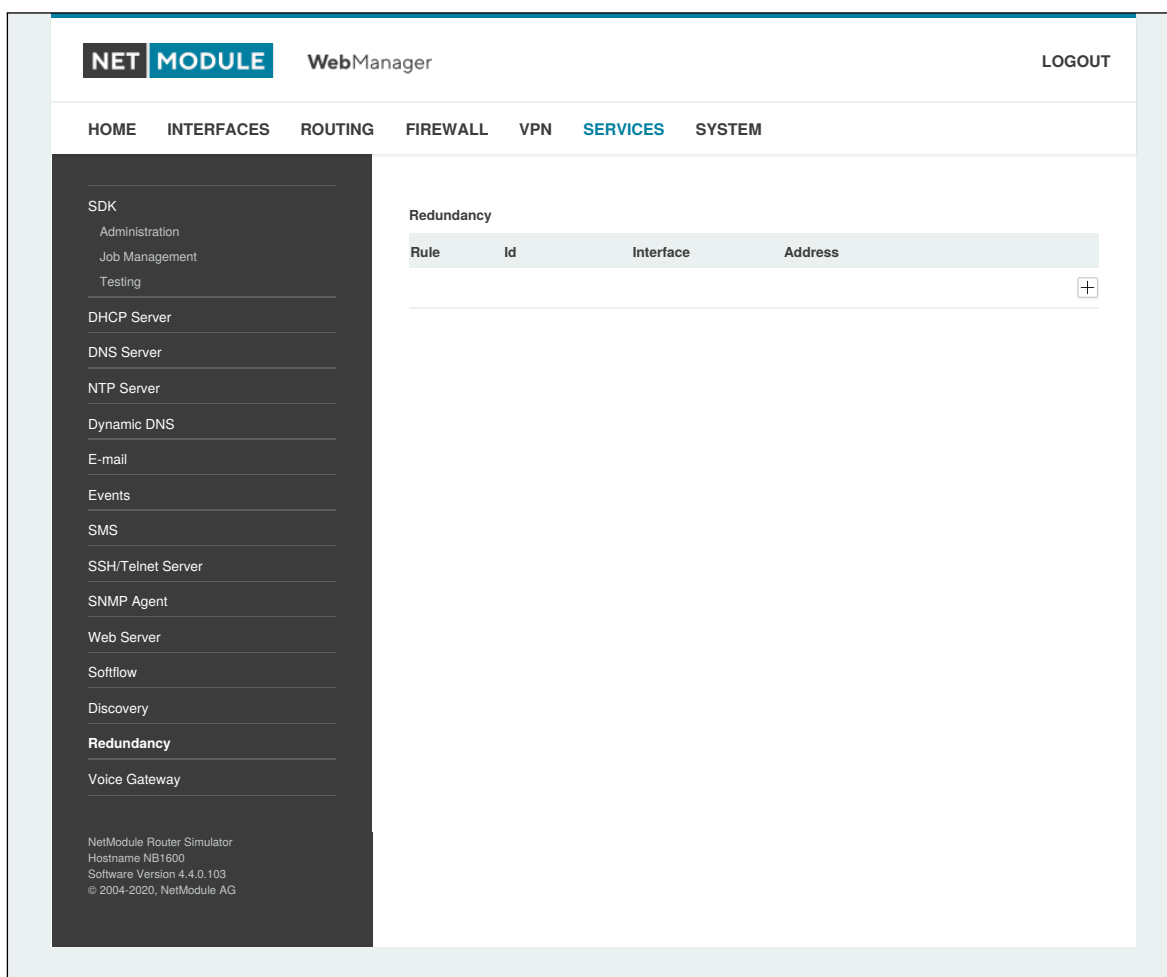
Abbildung 5.53.: VRRP-Konfiguration
