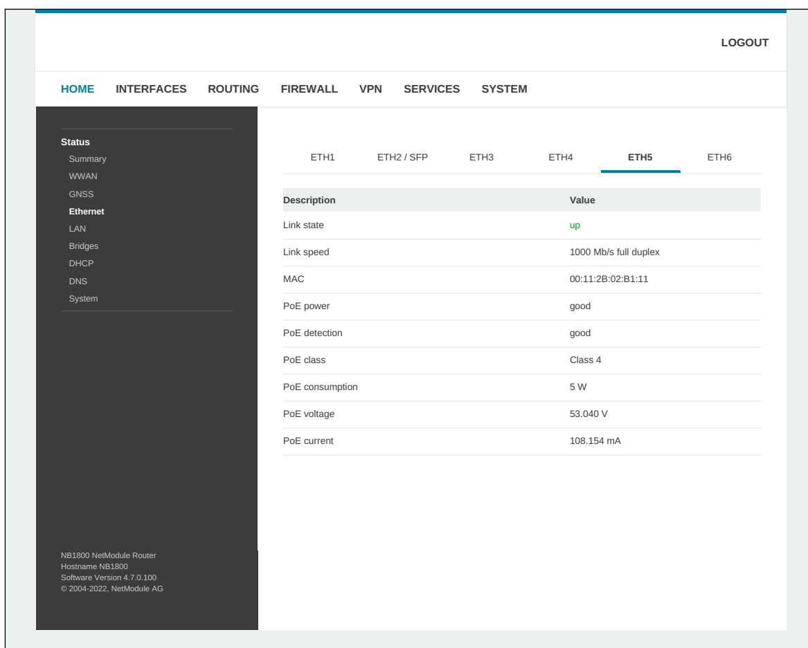
Abbildung 5.3.: Status des PoE-Power-Supply
