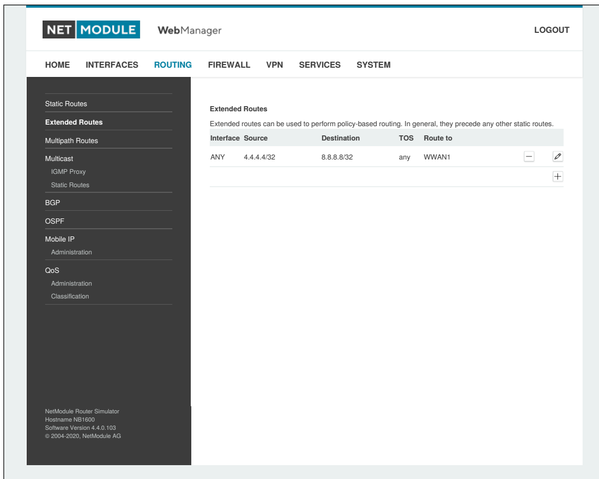
Abbildung 5.23.: Erweitertes Routing
