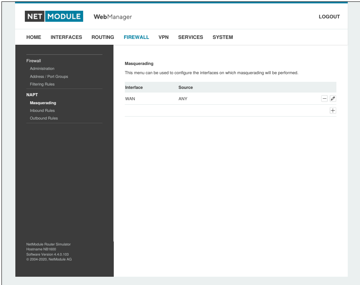
Abbildung 5.31.: Maskierung (Masquerading)
