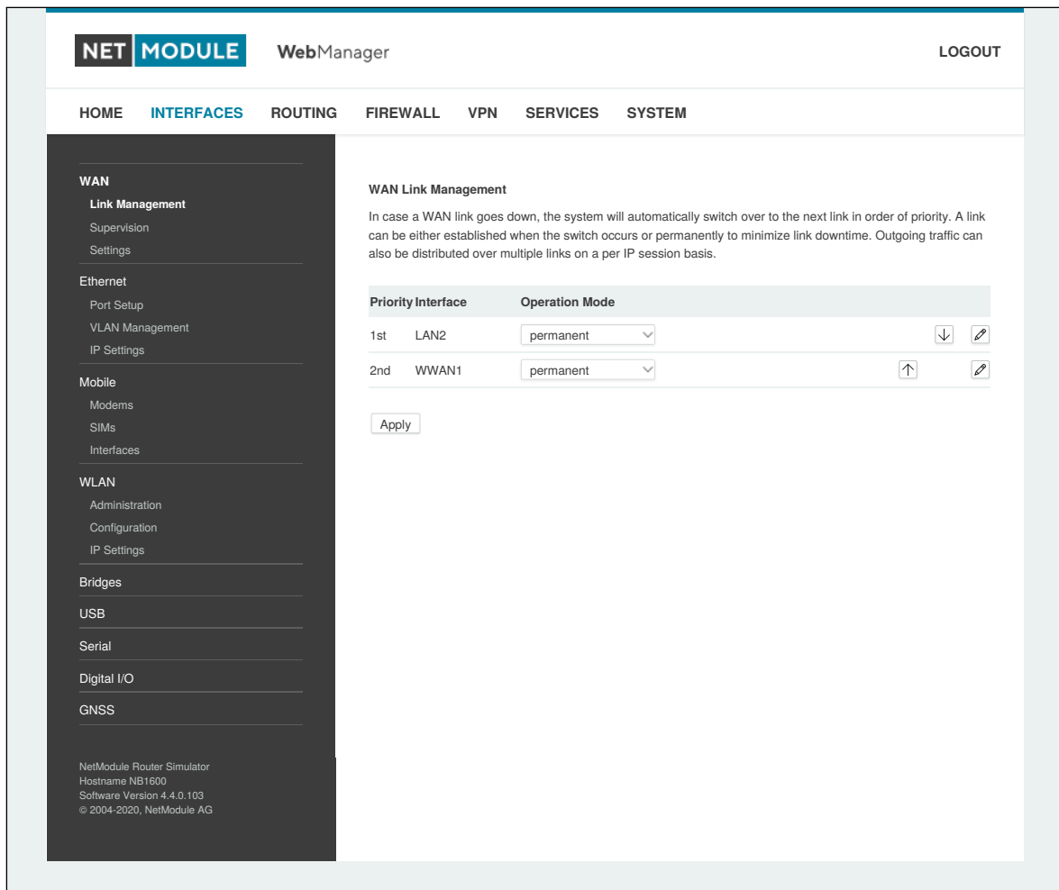
Abbildung 5.4.: WAN-Verbindungen
