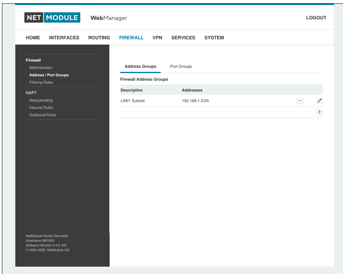
Abbildung 5.30.: Firewall-Gruppen
