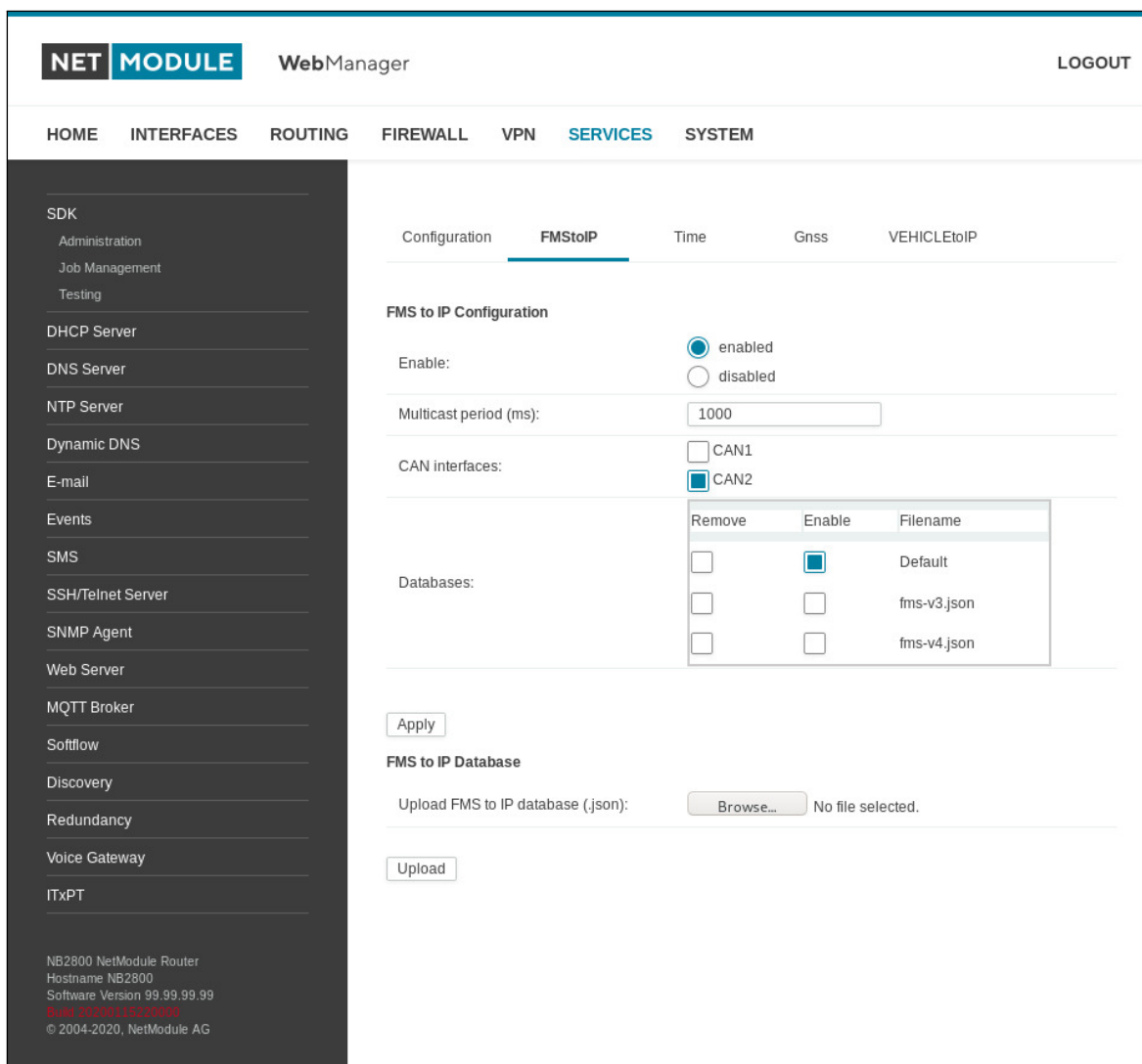
Abbildung 5.56.: ITxPT FMS-to-IP
