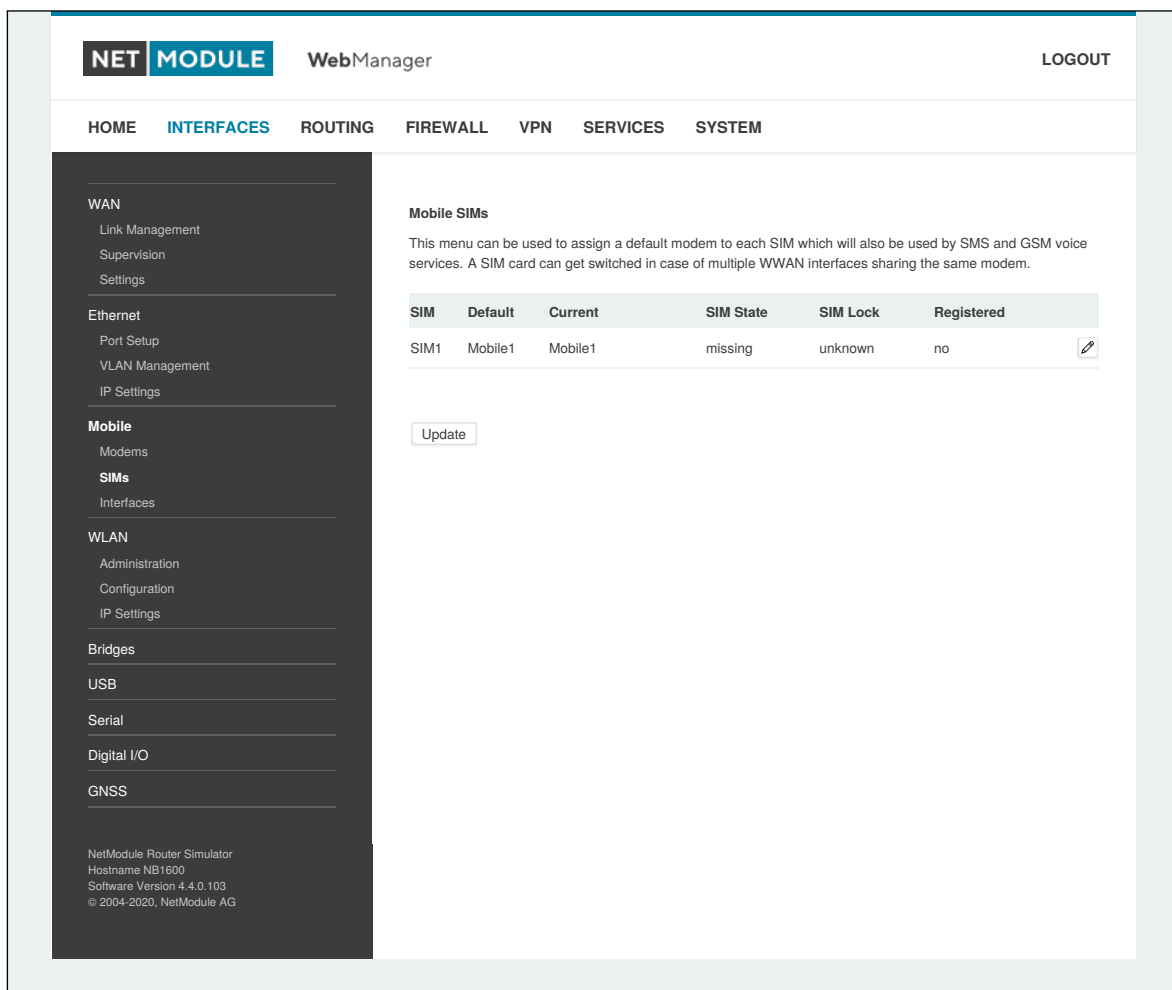
Abbildung 5.15.: SIM-Karten
